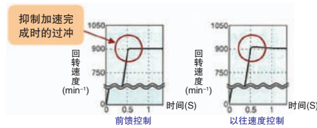
● 过冲比较
