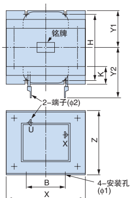
外形图2
