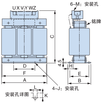
外形图1
