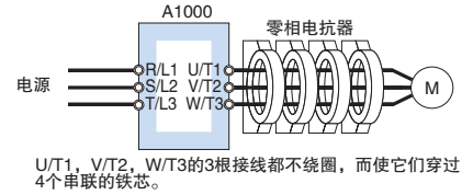
接线图b
