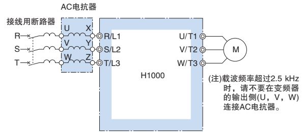
接线图
