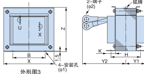
外形图3
