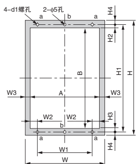
面板加工图1
