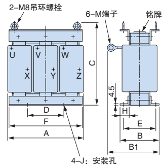
外形图3
